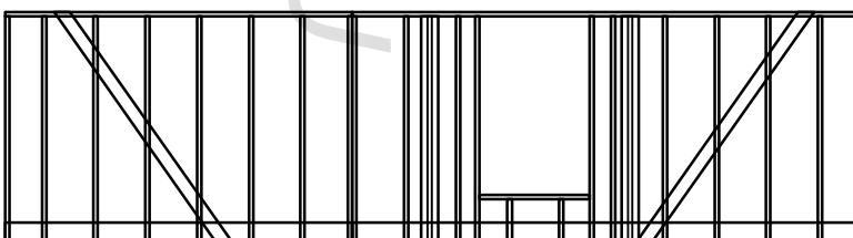
Рама 6-1
