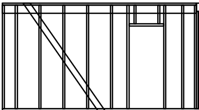
Рама 3-1
