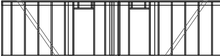
Рама 9-1
