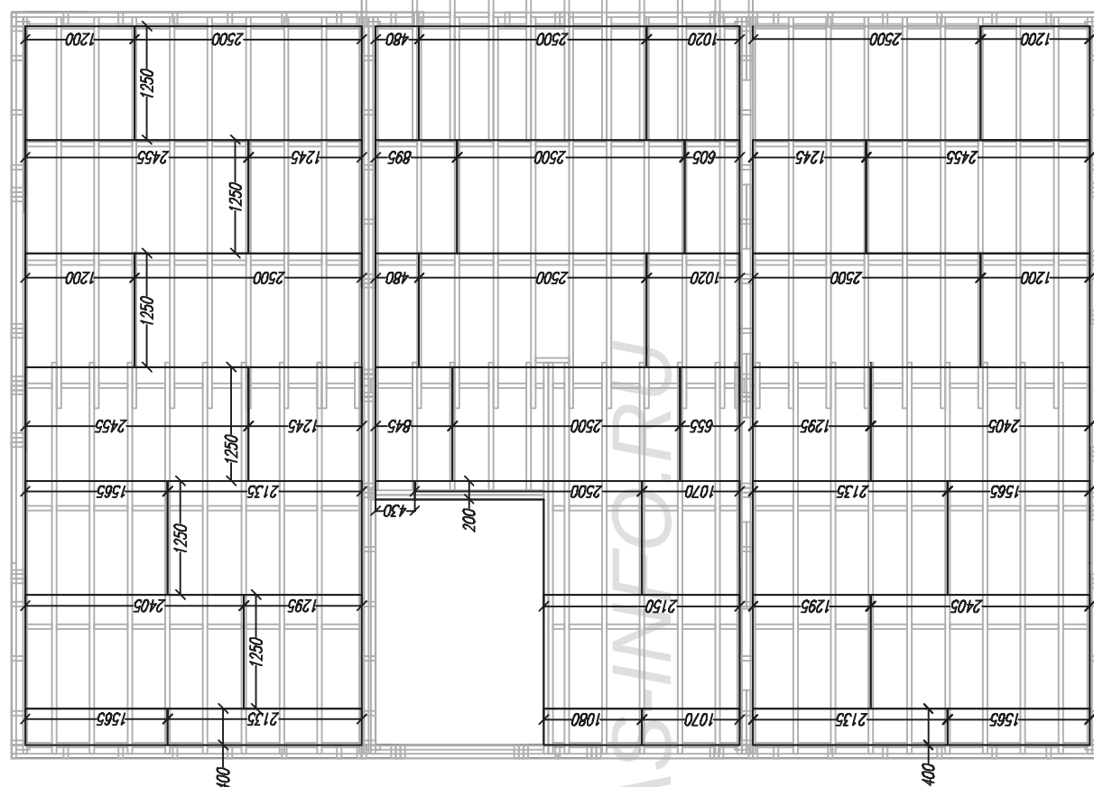
ПЛАН НАСТИЛА ОСЬ ПЕРВОГО ЭТАЖА
