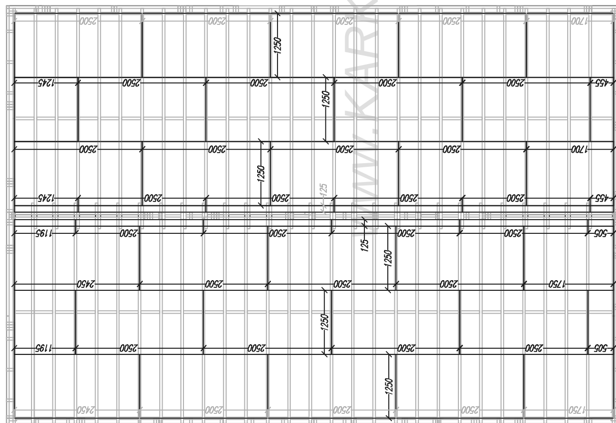
ПЛАН НАСТИЛА ОСЬ ПЕРВОГО ЭТАЖА
