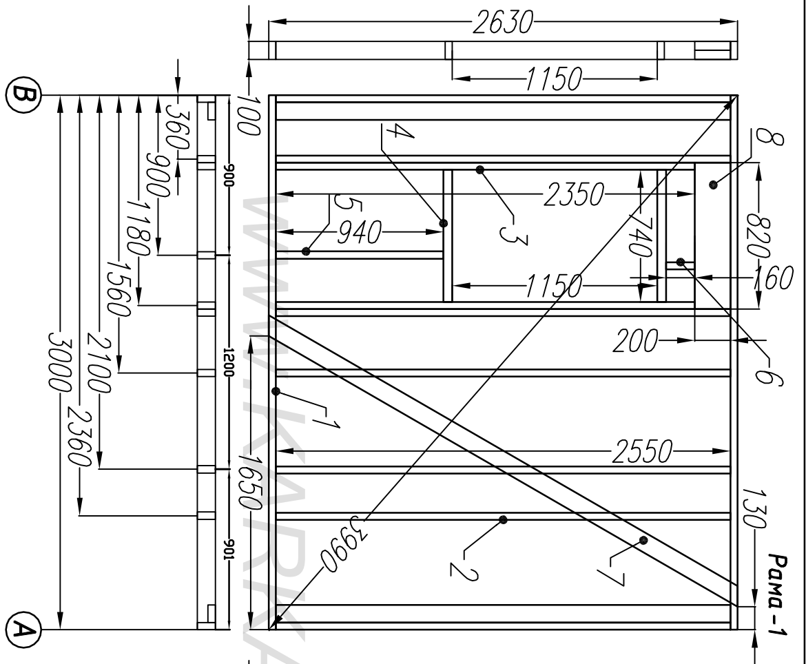
Раскрой: Рама-1.
